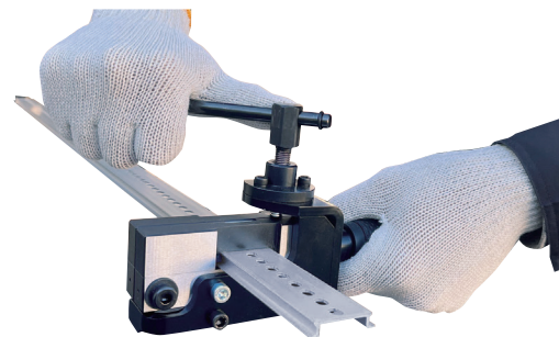
D11102 モクバ DIN レールカッター ハンディー スクリューホルダーセット
